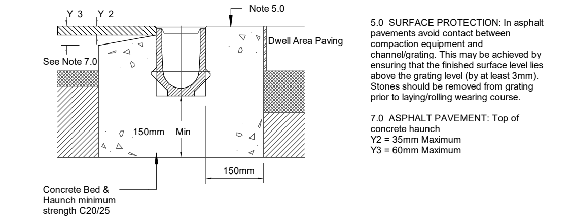
9 Aco Drain Section 1 : 10
