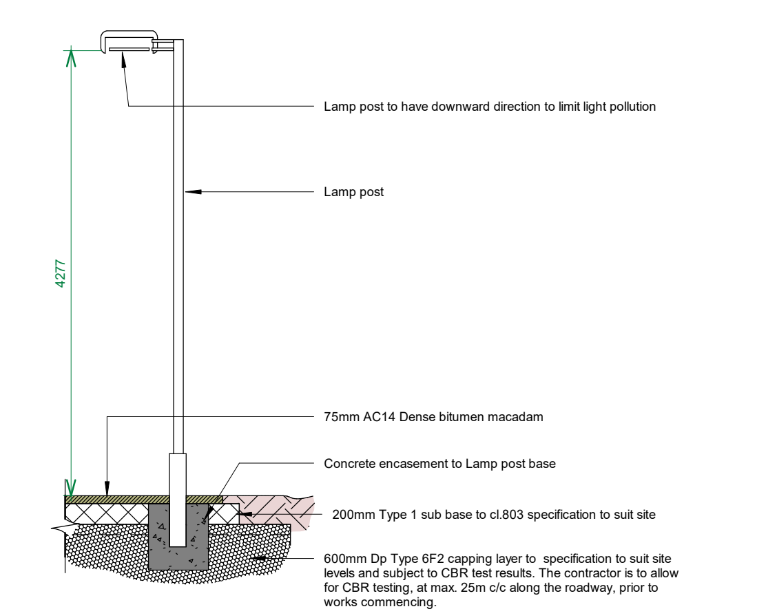
11 Lamp Post 1 : 50
