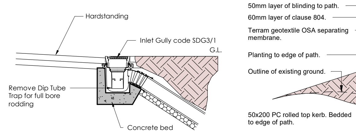
6 Inlet Gully 1 : 20
